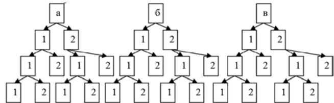
Рис. 4. Дерево аналитических решений ФКП Баркера
